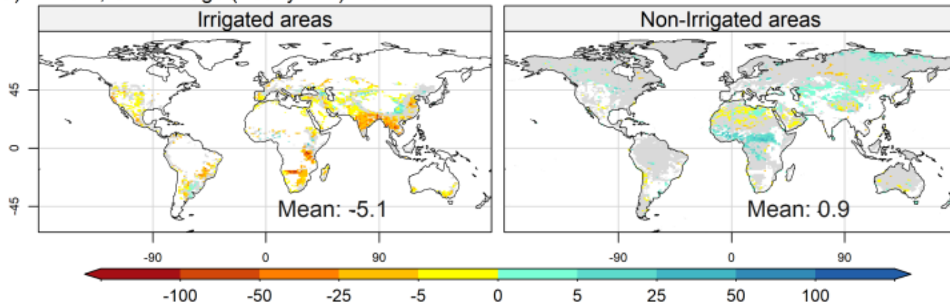
b) Irr-Nolrr, Stream storage (Yearly mm): Fut
