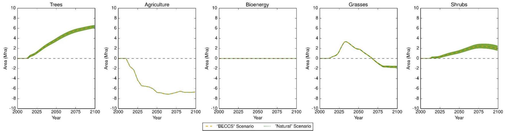
Fig. SI.2z: Oceania
