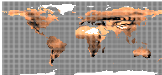
(d) PI carbon storage
