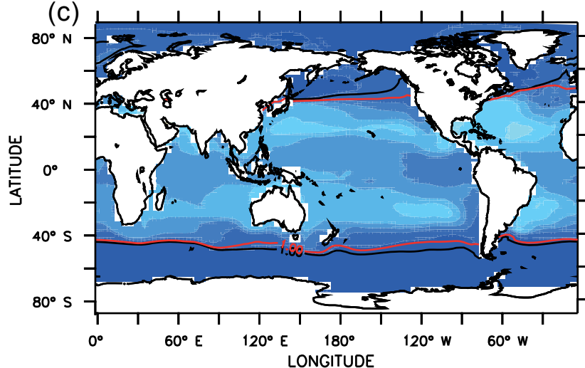
RCP8.5_AOA_ST
