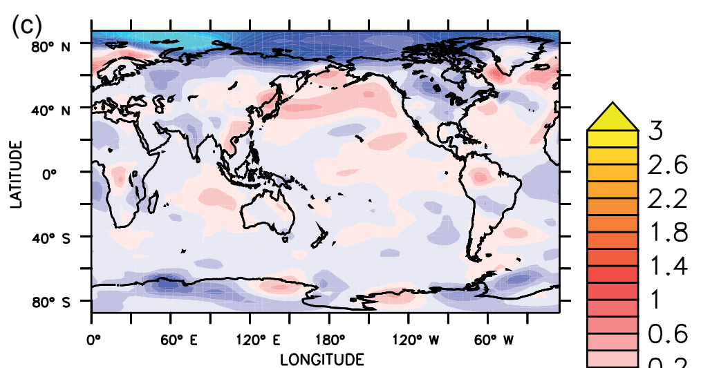
RCP8.5_AOA_ST
