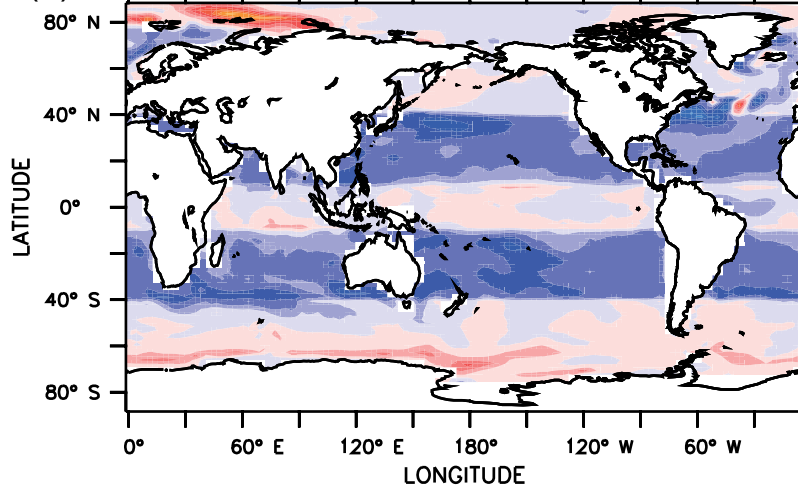
RCP8.5_AOA_ST
