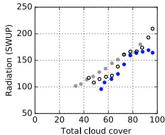
HadGEM2-A HadGEM3-A
