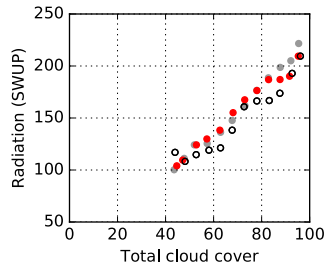
MPI-ESMnoembrace MPI-ESMwithembrace
