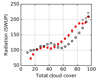
MPI-ESMnoembrace MPI-ESMwithembrace
