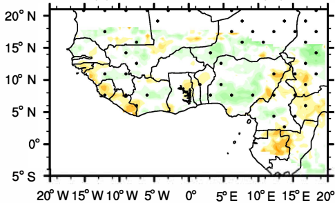
(d) Grell minus GPCP (%)
