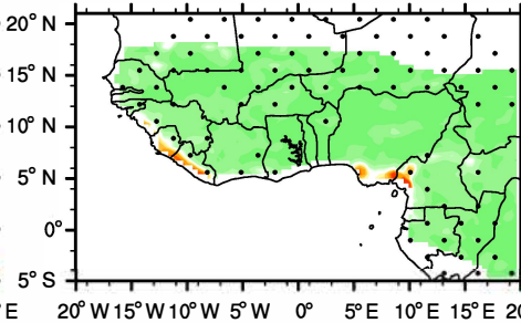
(e) Tiedtke minus GPCP (%)
