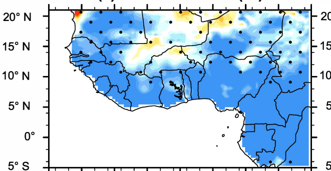
(d) Grell minus CRU ( ^{\circ}\text{C} )
