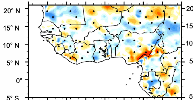
(a) UDEL minus CRU ( ^{\circ}\text{C} )
