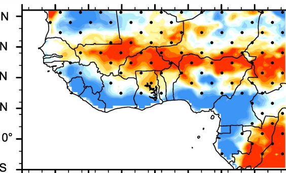
(e) Tiedtke minus CRU ( ^{\circ}\text{C} )
