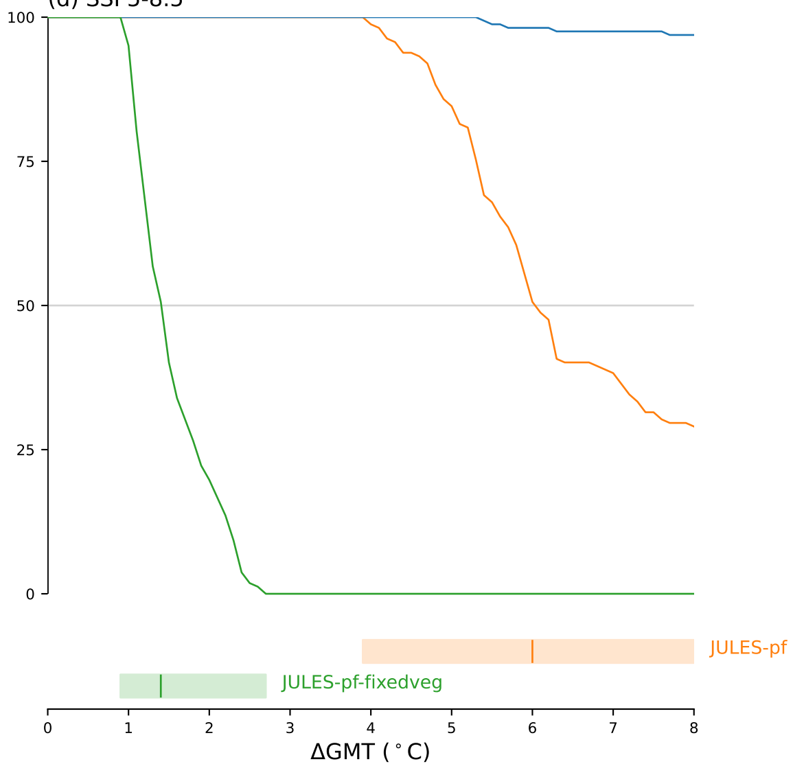
(d) SSP5-8.5
