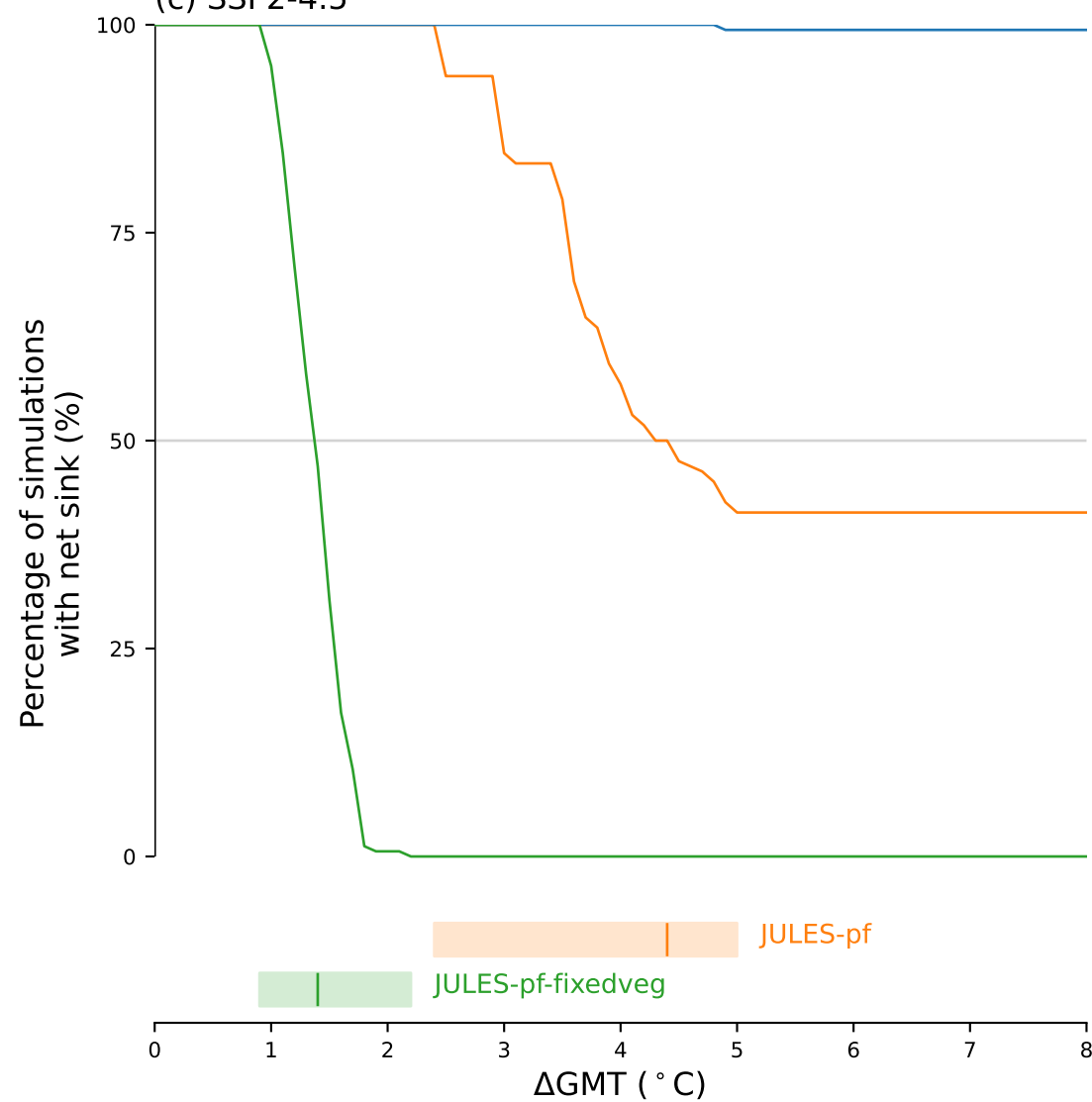
(c) SSP2-4.5
