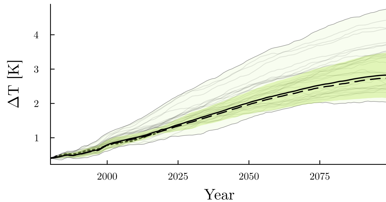
ssp245
