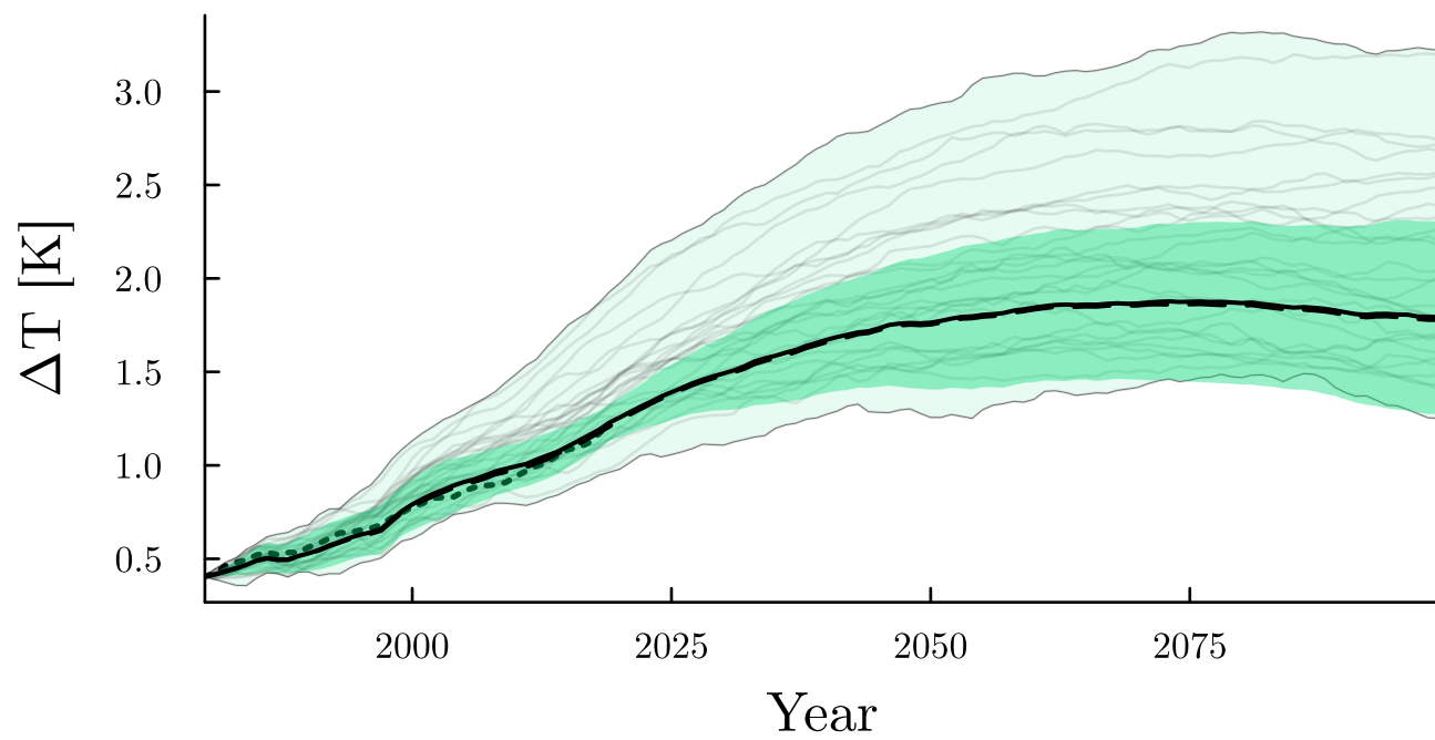
ssp126
