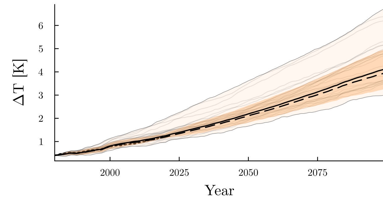
ssp370
