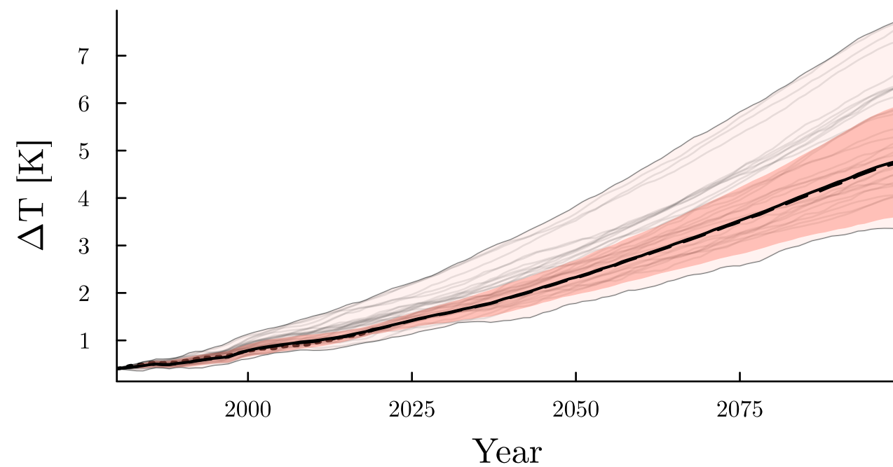
ssp585
