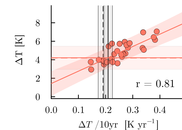
ssp585, 2090
