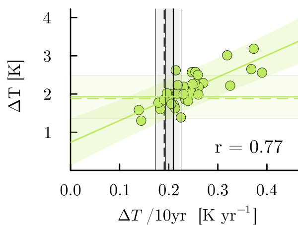
ssp245, 2050
