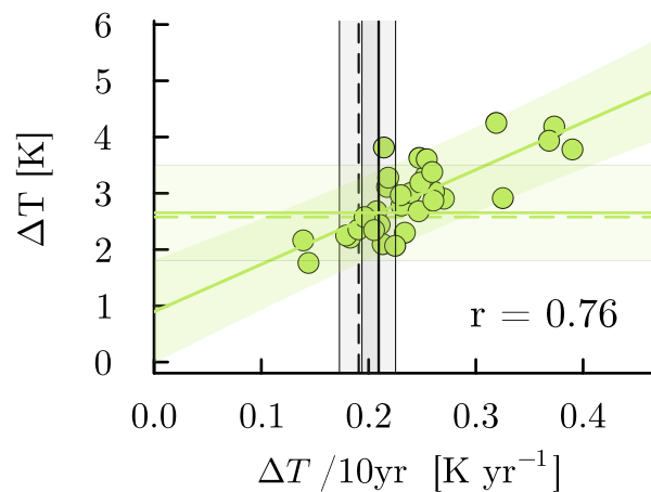
ssp245, 2090
