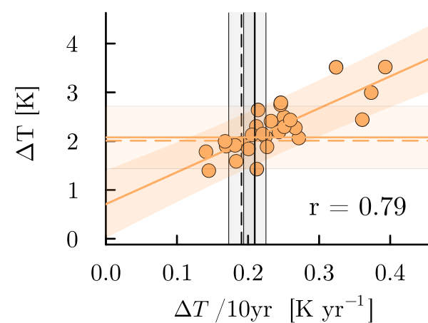
ssp370, 2050
