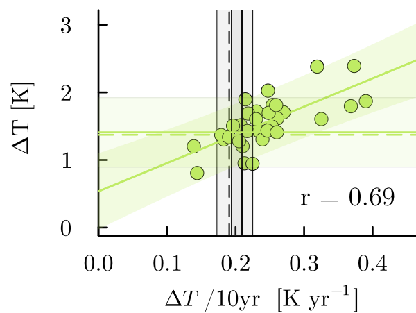
ssp245, 2030
