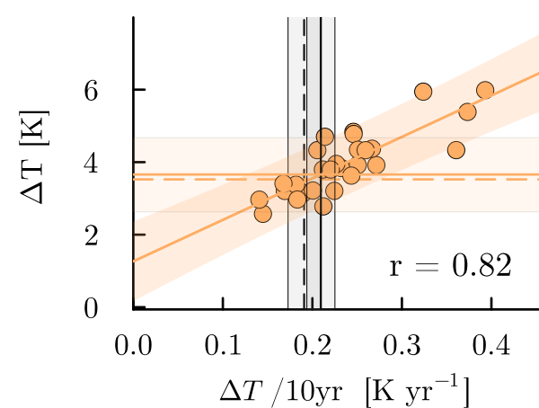
ssp370, 2090
