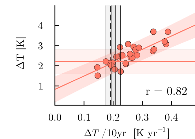
ssp585, 2050
