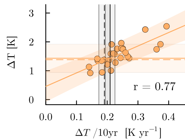
ssp370, 2030
