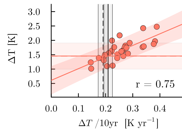
ssp585, 2030
