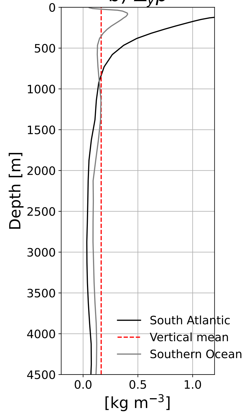
b) \Delta_y \rho
