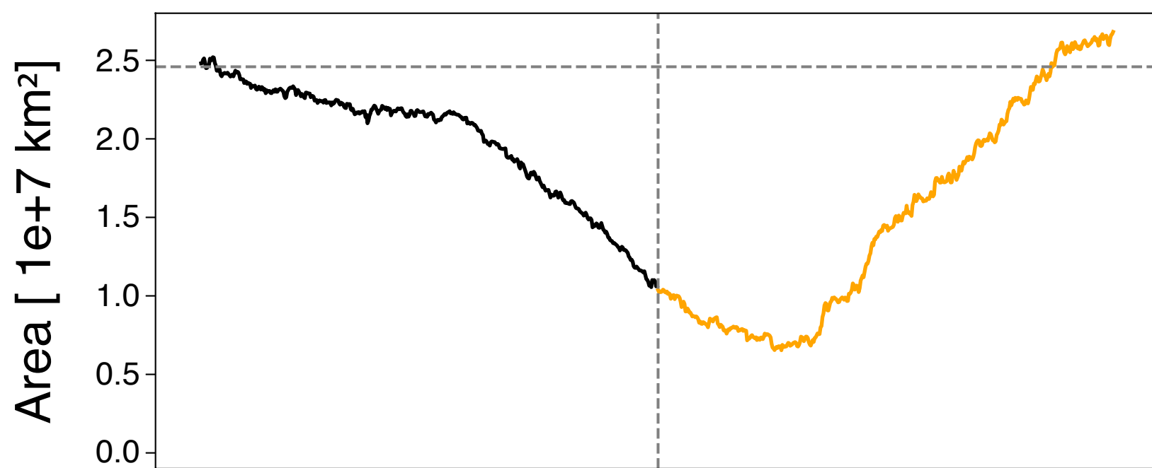
Permafrost Area
