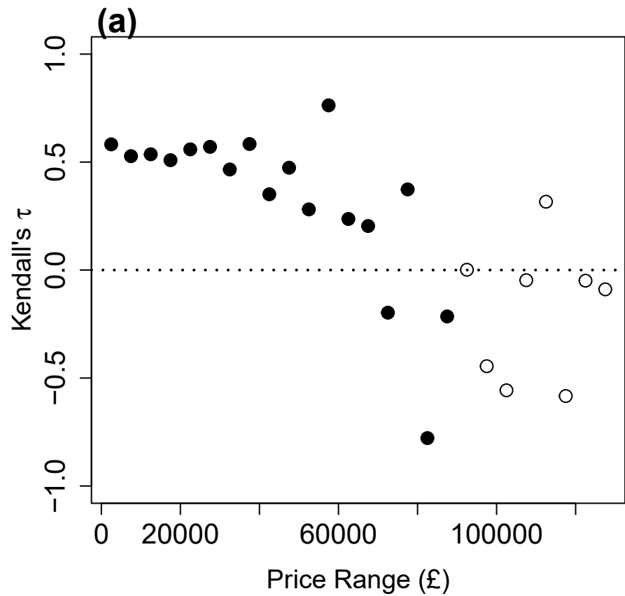
AR(1)
