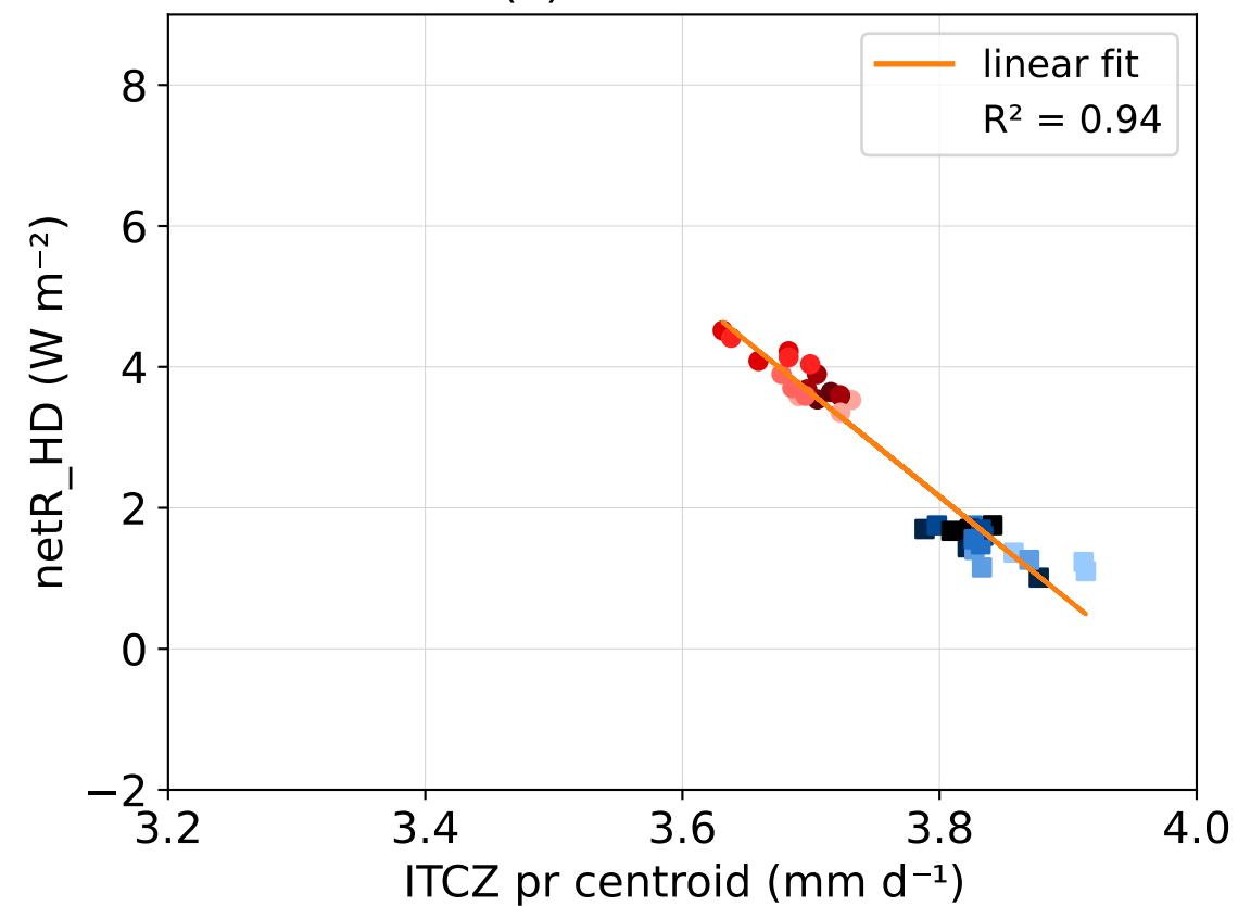
(d) UKESM1-0-LL
