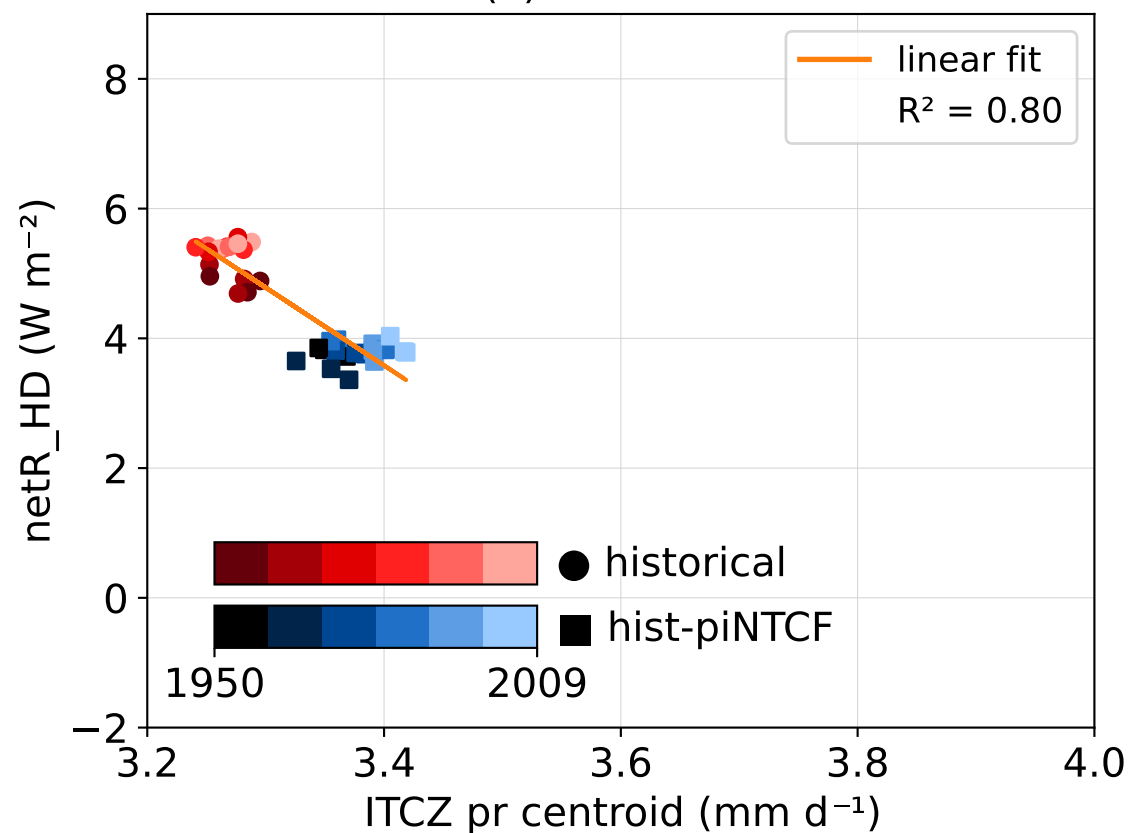
(a) BCC-ESM1
