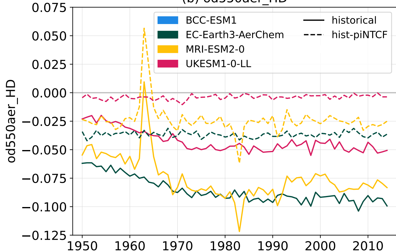
(b) od550aer_HD
