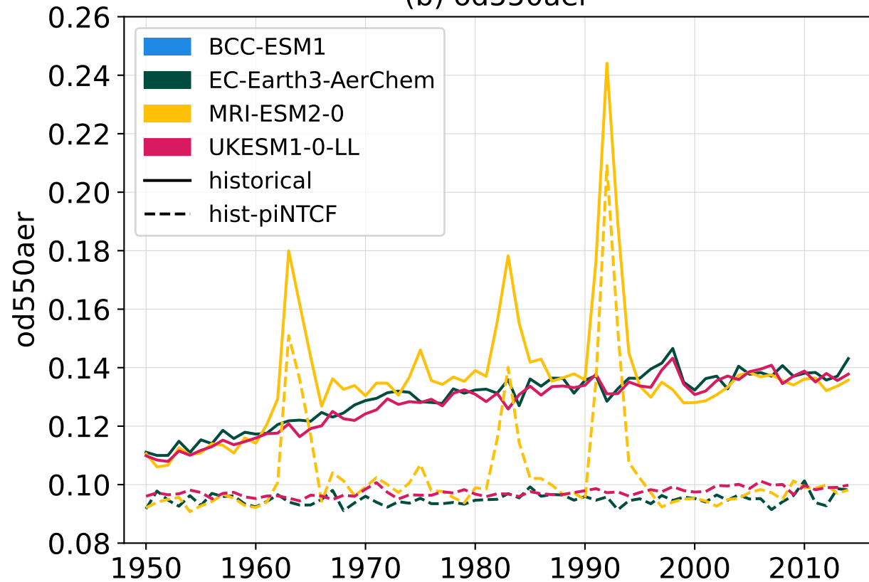
(b) od550aer
