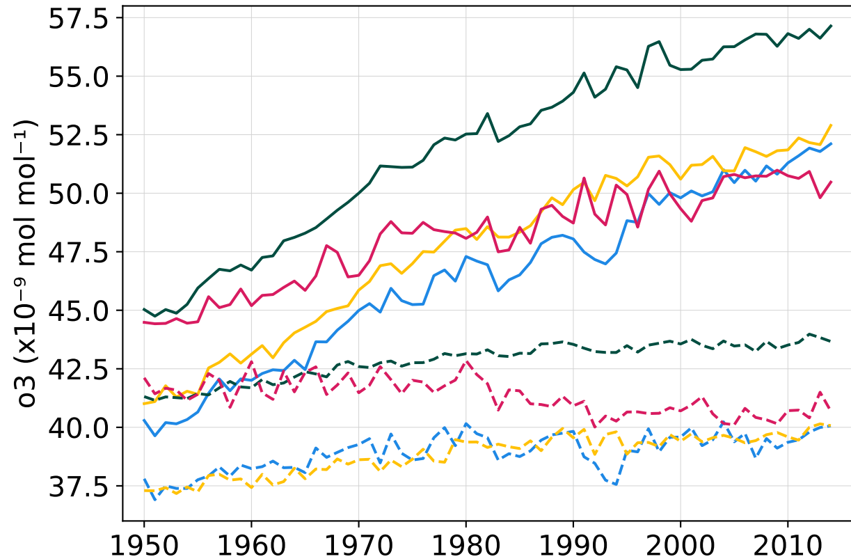
(a) o3
