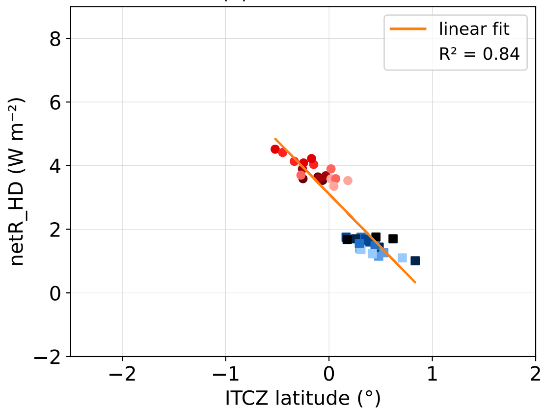
(d) UKESM1-0-LL
