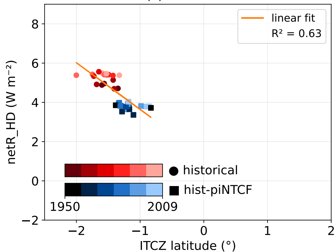
(a) BCC-ESM1
