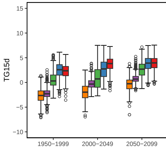
(d) SSP5-8.5
