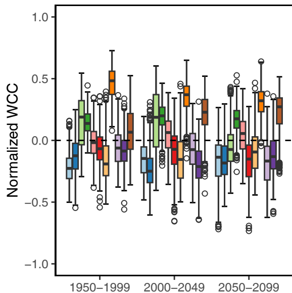
(a) SSP1-2.6
