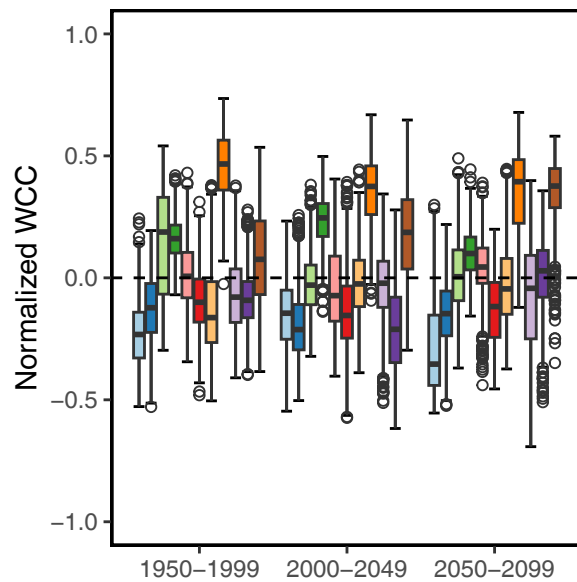
(d) SSP5-8.5
