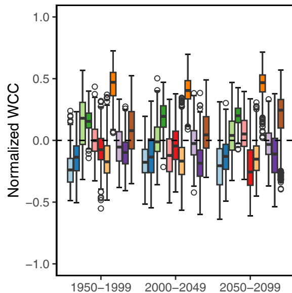
(b) SSP2-4.5
