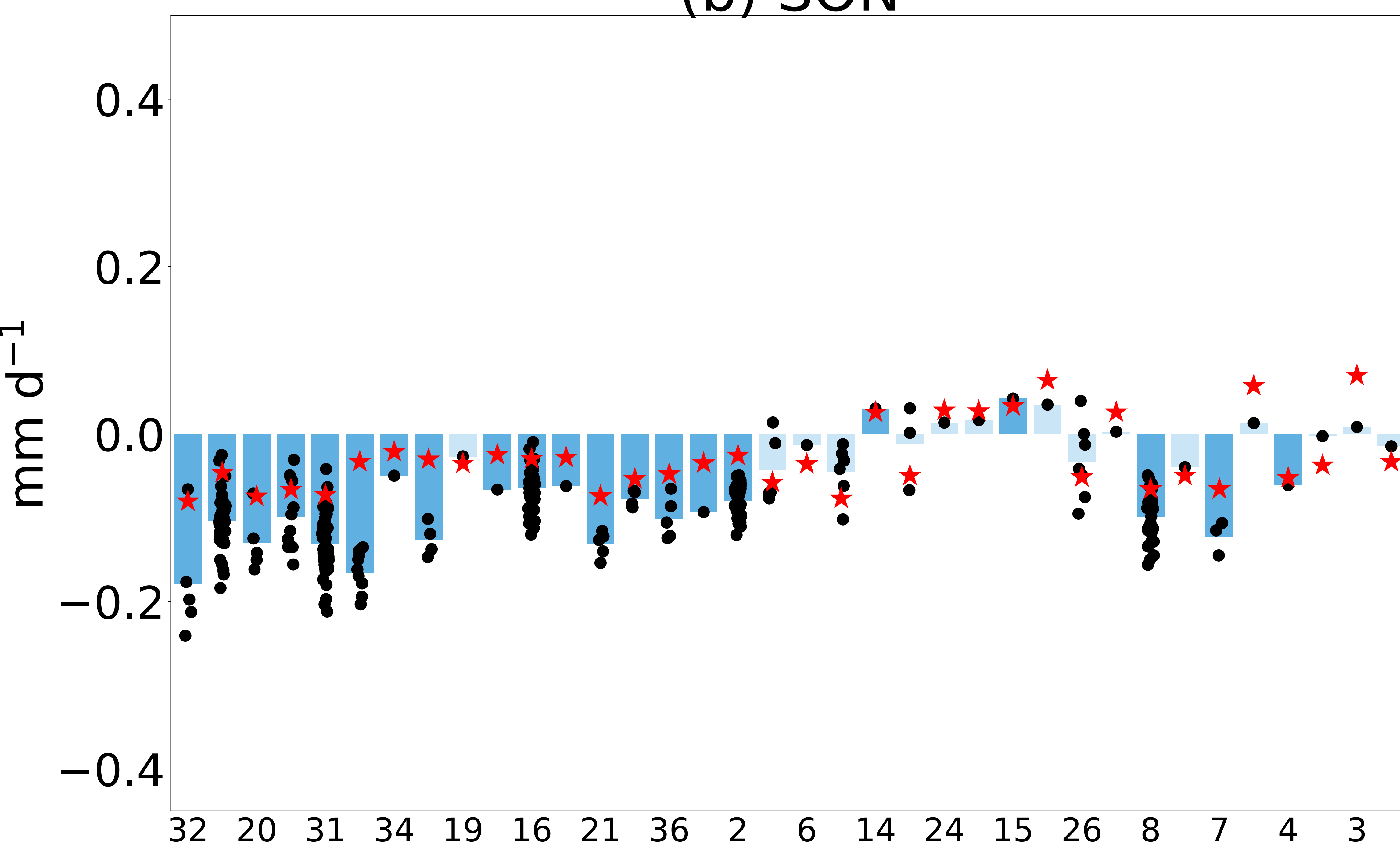
(b) SON
