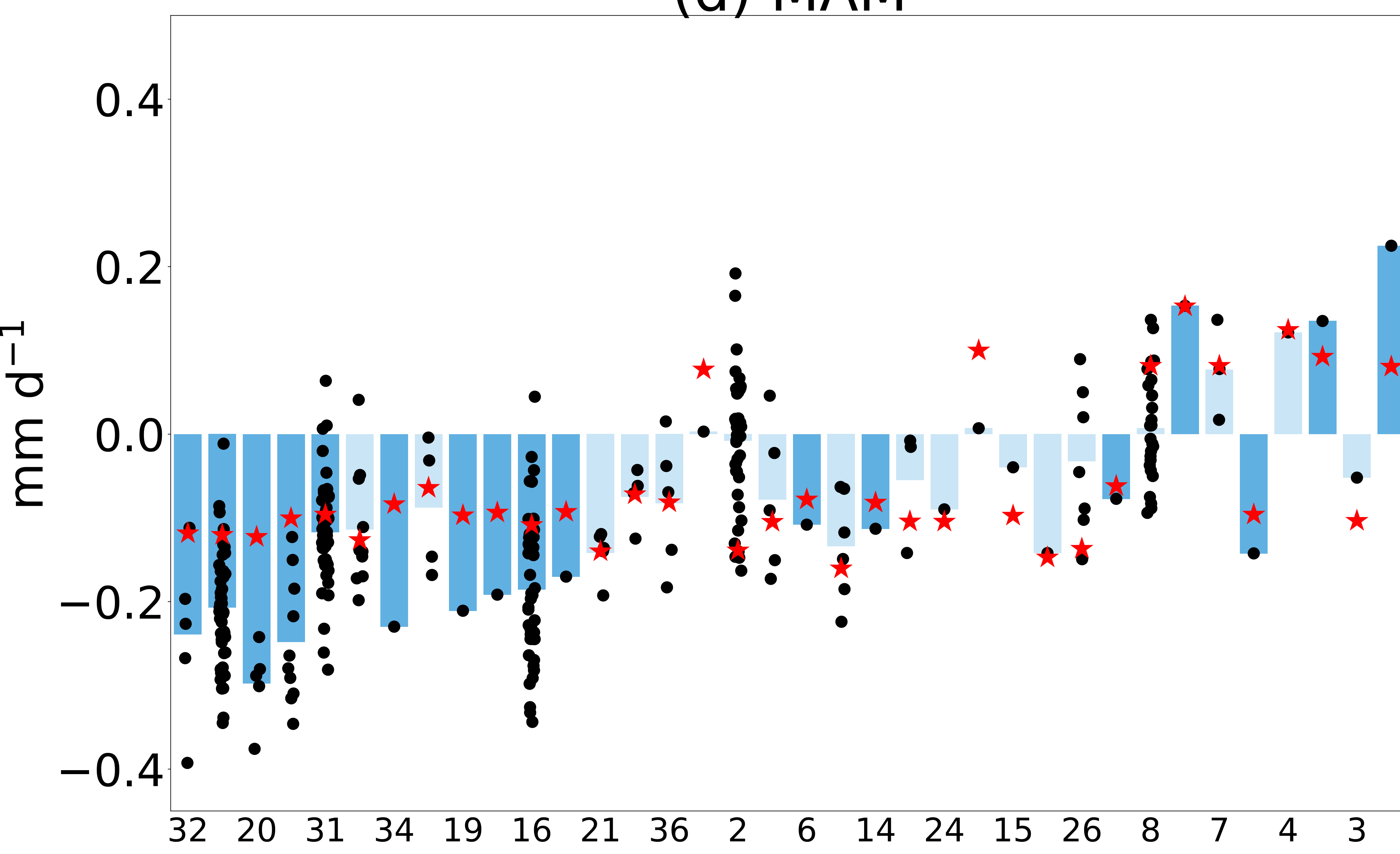
(d) MAM
