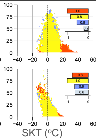
MERRA-2
