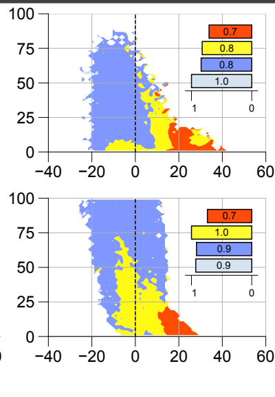
ERA5/CAMS4
