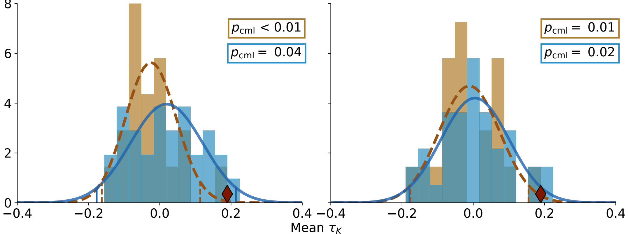
MIROC-ES2L
