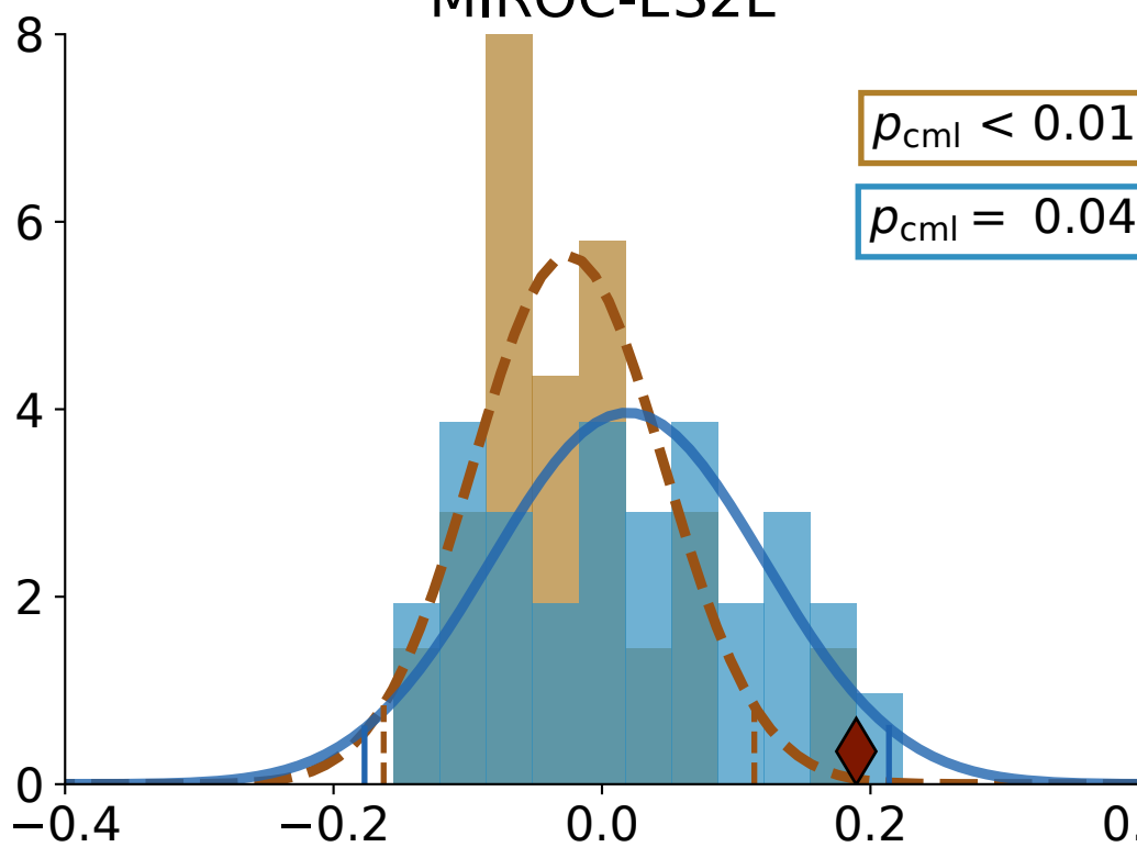
MIROC-ES2L
