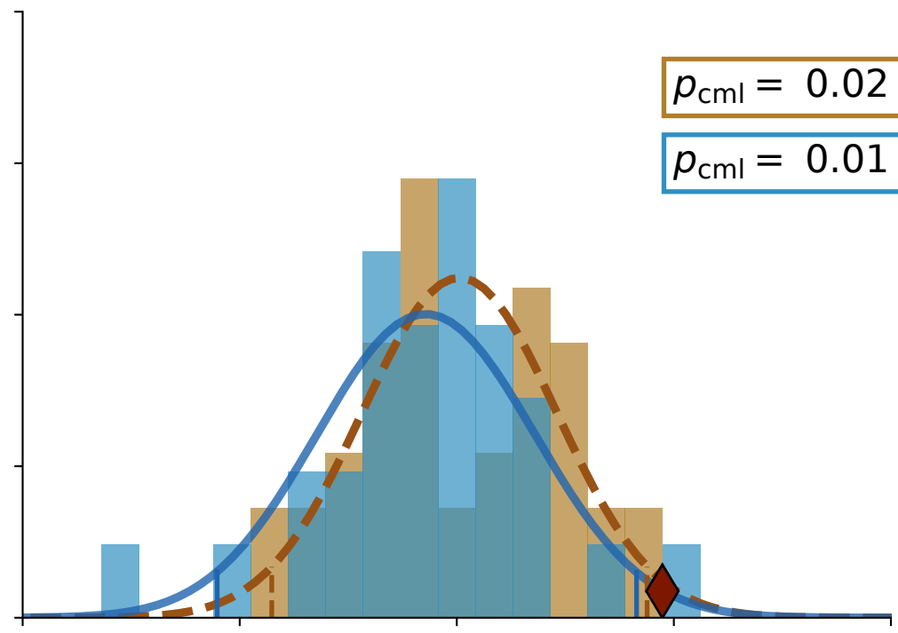
MPI-ESM1-2-LR
