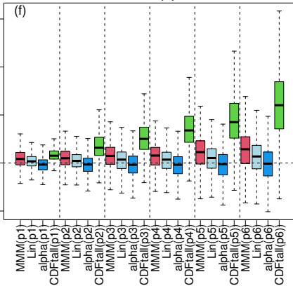
Bmax(T)
