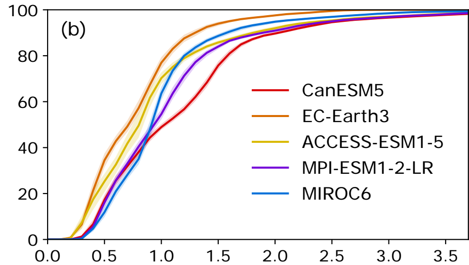
TNx
