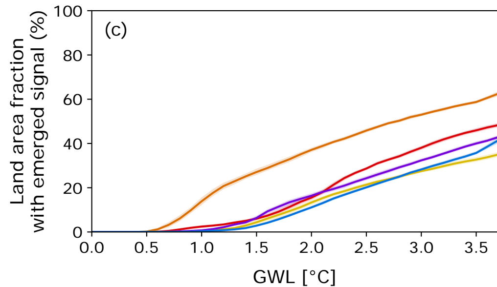
PRCptot
