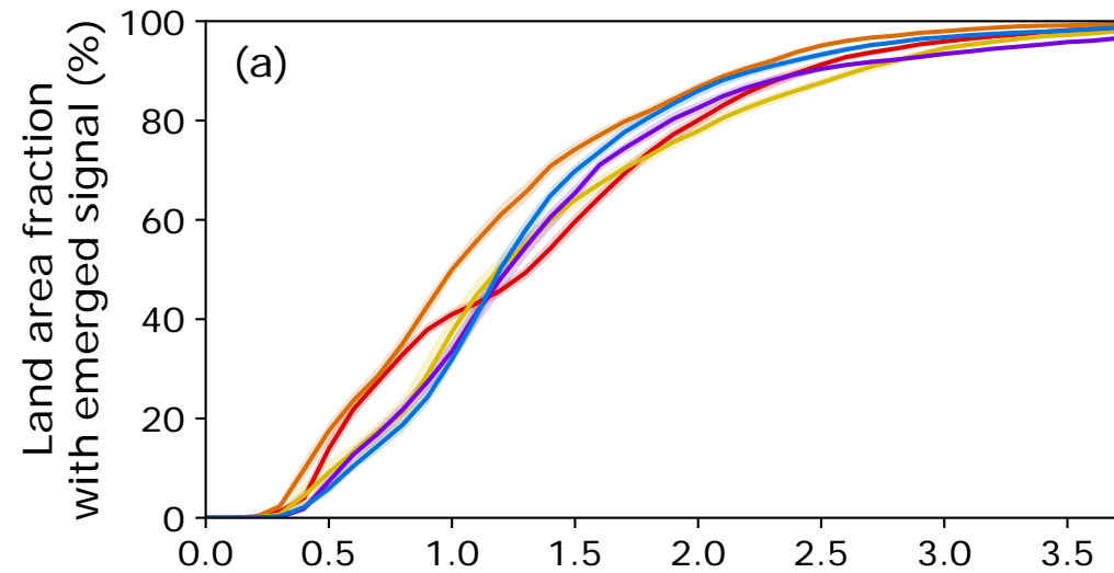
TXx
