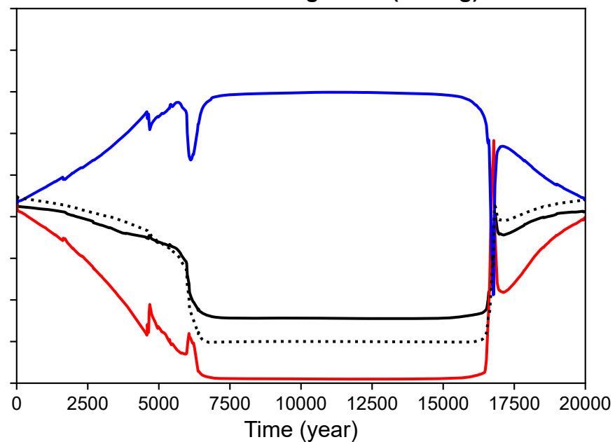
(d) Thermal wind diagnostic (hosing)
