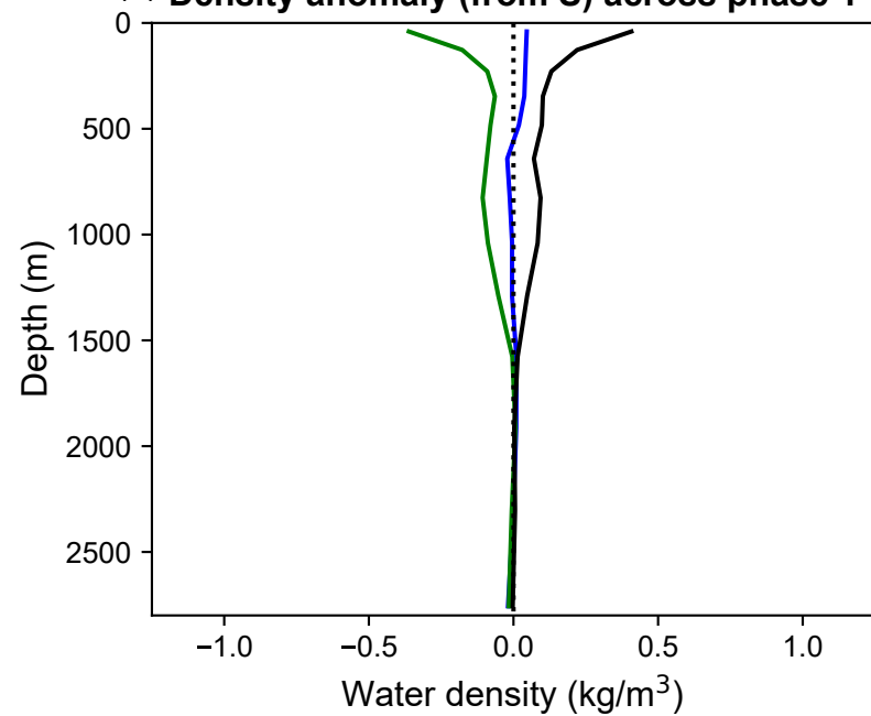
(d) Density anomaly (from S) across phase 1
