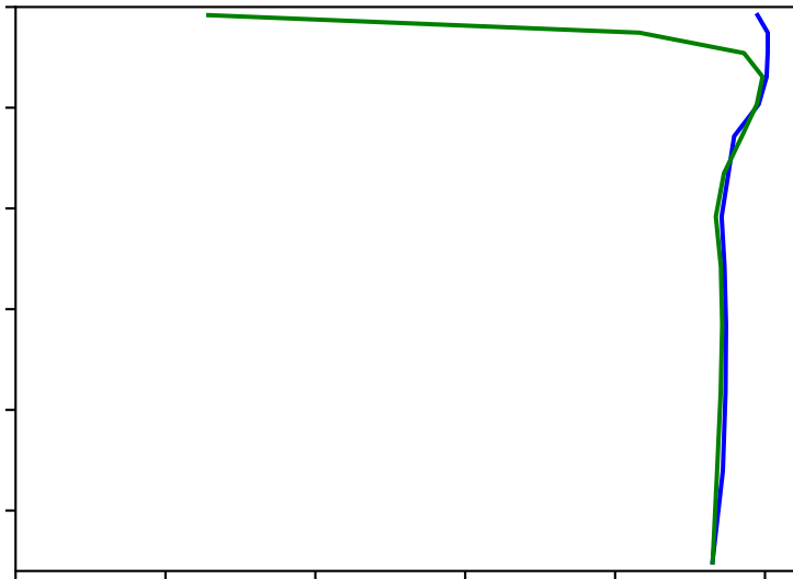
(d) Vertical salinity (PSU) profile at year 2100
