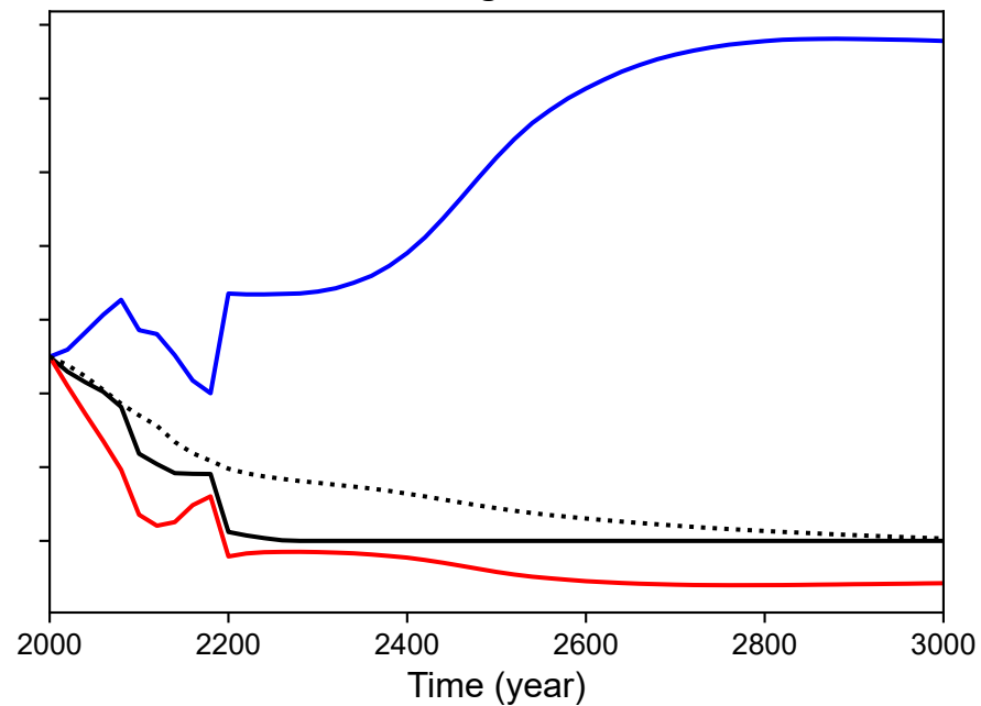
(d) Thermal wind diagnostic above 30 ^{\circ} N
