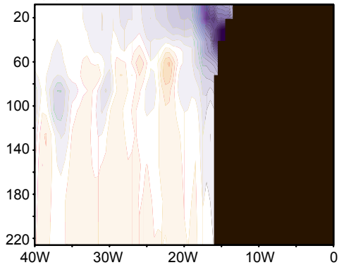
(d) Dakar Niña, ROM F
