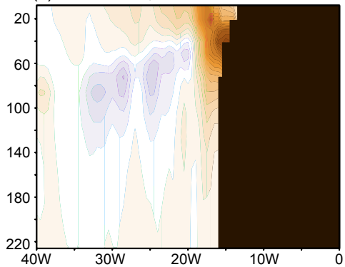
(c) Dakar Niño, ROM F
