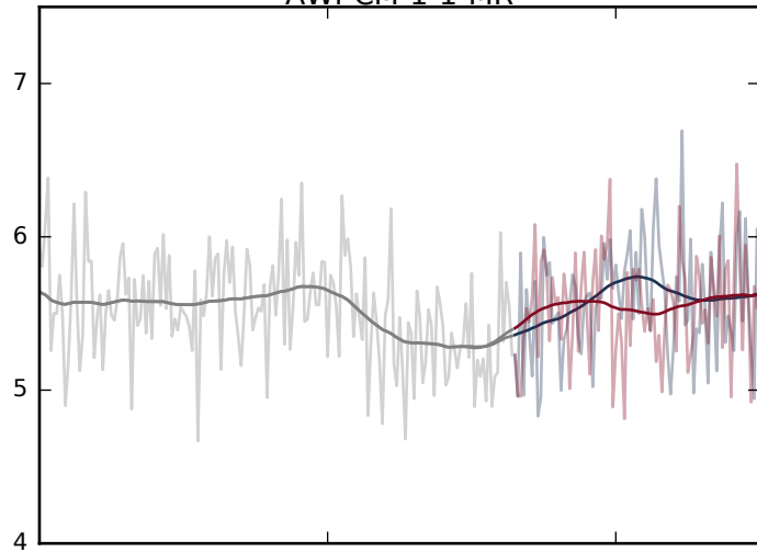
AWI-CM-1-1-MR
