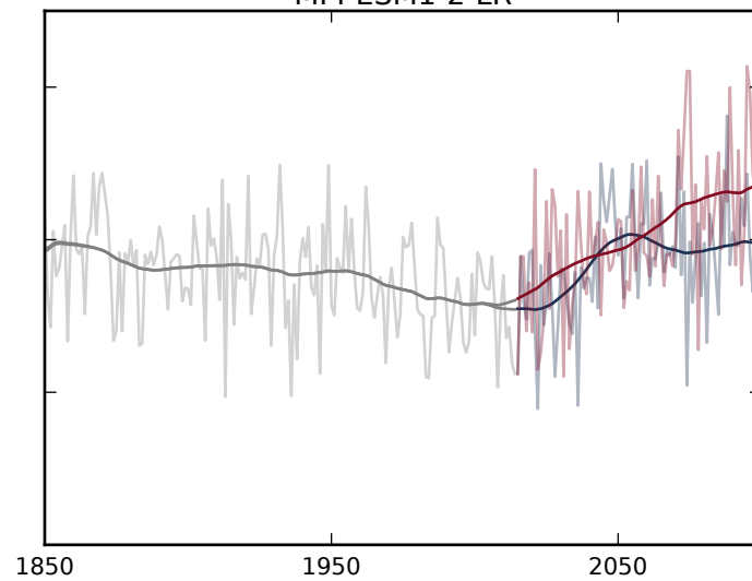
MPI-ESM1-2-LR
