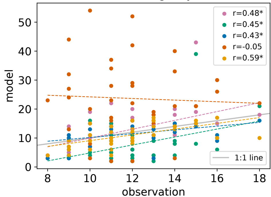
(d) GPP lag (days)
