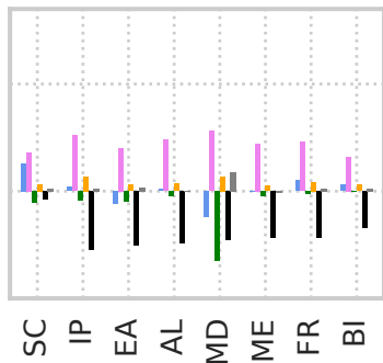
(d) OLR JJA
