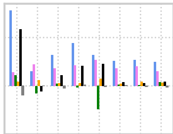
(d) OLR JJA
