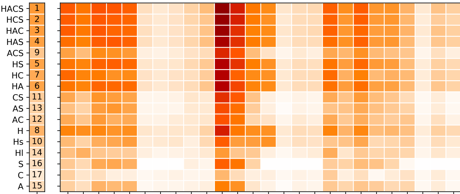
MPI-ESM1-2-LR
