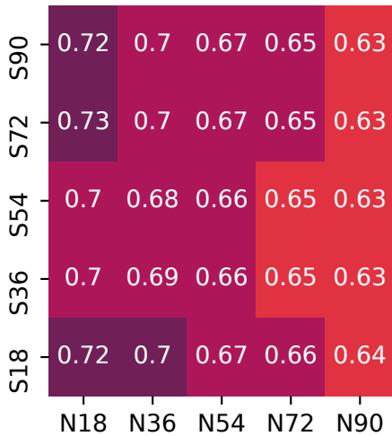
AGR_R
