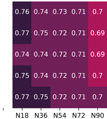
SL_{Resid}
