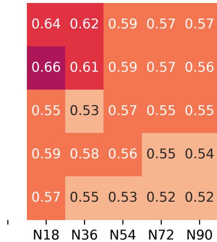
SL_{DGVMs}
