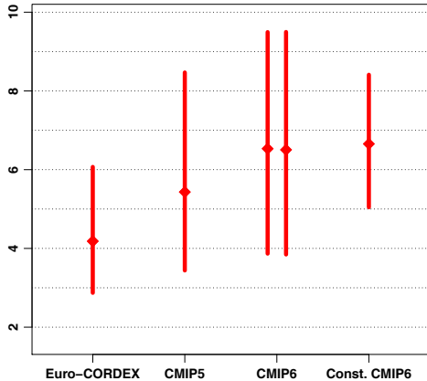
Summer (JJA)
