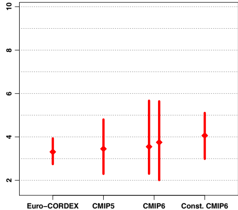
Winter (DJF)
