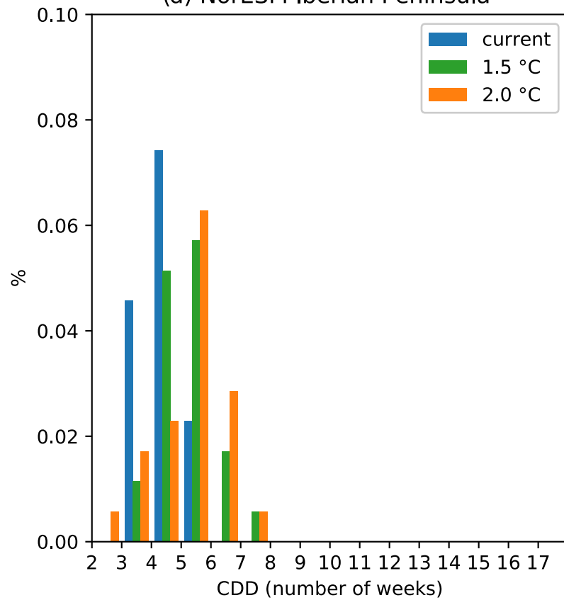
(d) NorESM Iberian Peninsula
