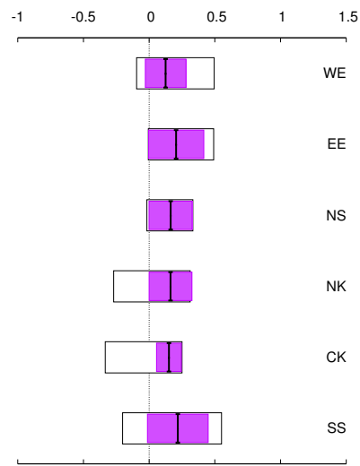
(d) Evaporative Demand
