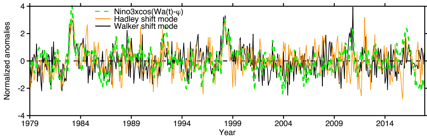
(b) Nino3 vs WC2&HC1 [OBS]
