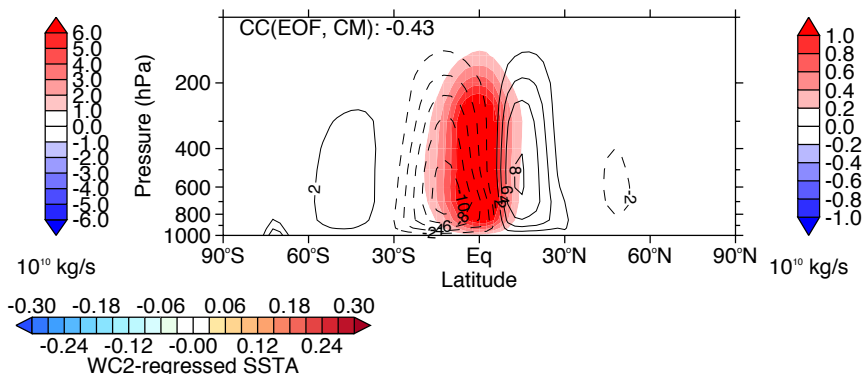
(b) EOF 1, Hadley shift mode, ERAI (30.19 %)
