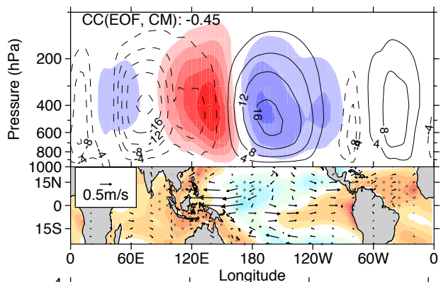
(a) EOF 2, Walker shift mode, ERAI (18.05 %)
