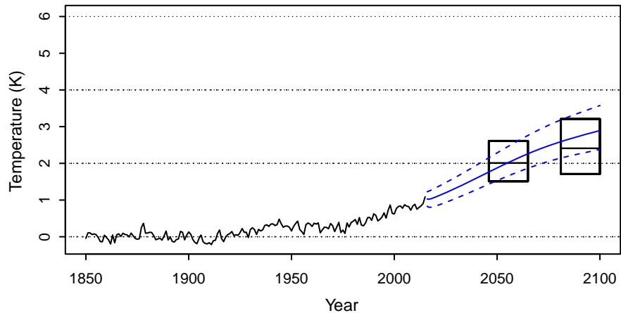
(d) RCP8.5 (scaling)
