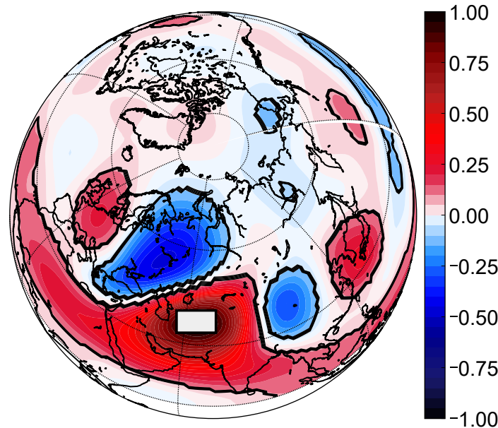
(d) Lag-0 correlation of Z200 with CGTI
