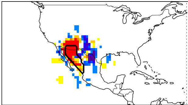
(b) E-P anom (ext-low) JA Day -2
